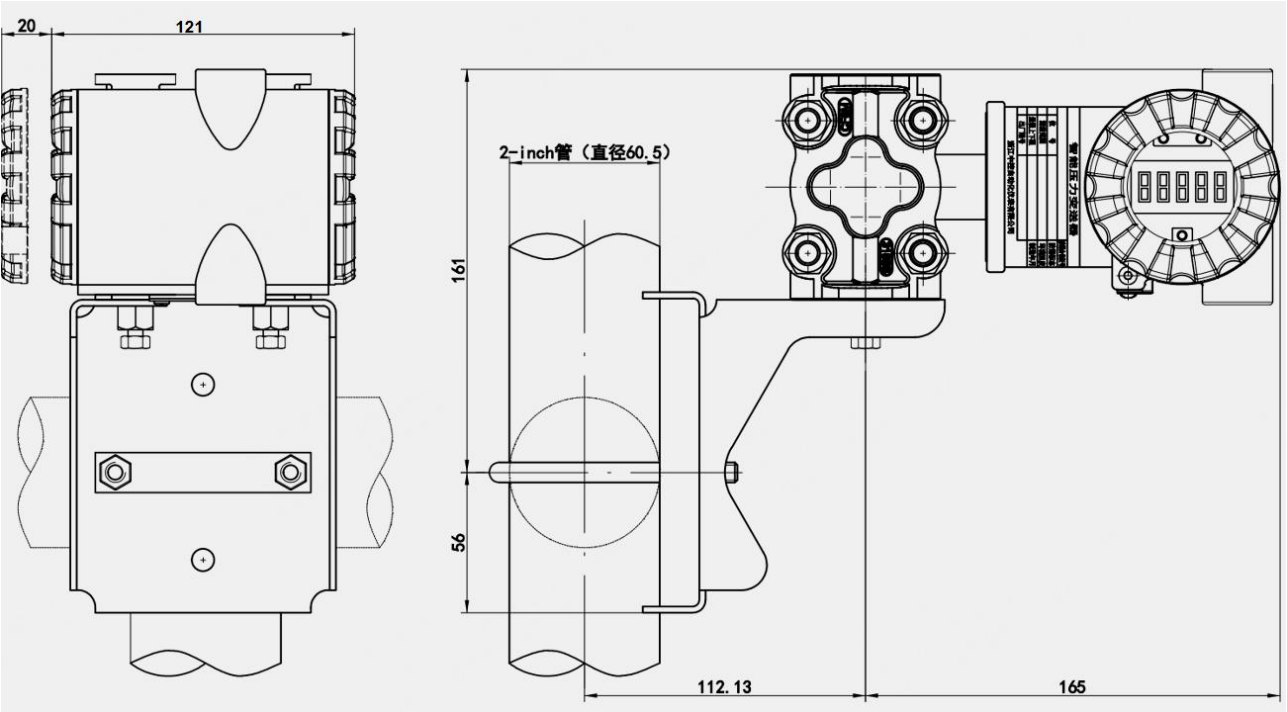
垂直配管连接图（板装弯支架）
