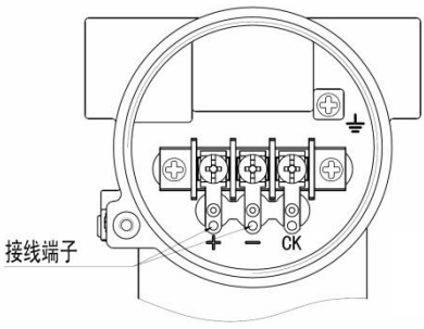
端子侧接线图
