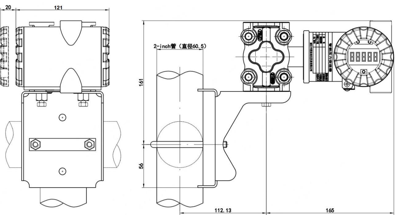
垂直配管连接图 (管装弯支架)
