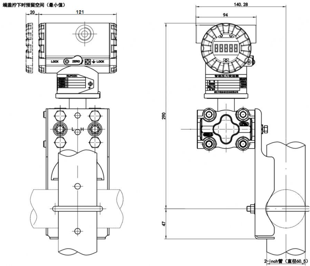
水平配管连接图（管装平支架）
