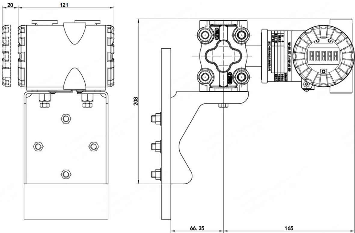
水平配管连接图（管装平支架）
