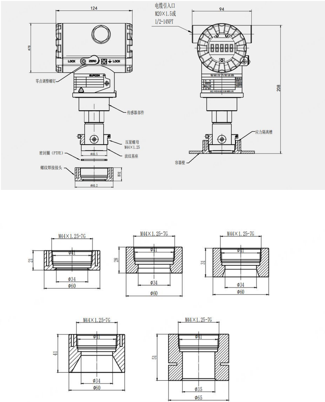
M44*1.25 接口示意图:
