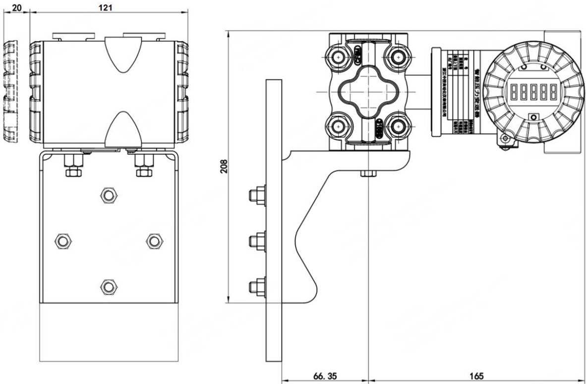
垂直配管连接图（板装弯支架）
