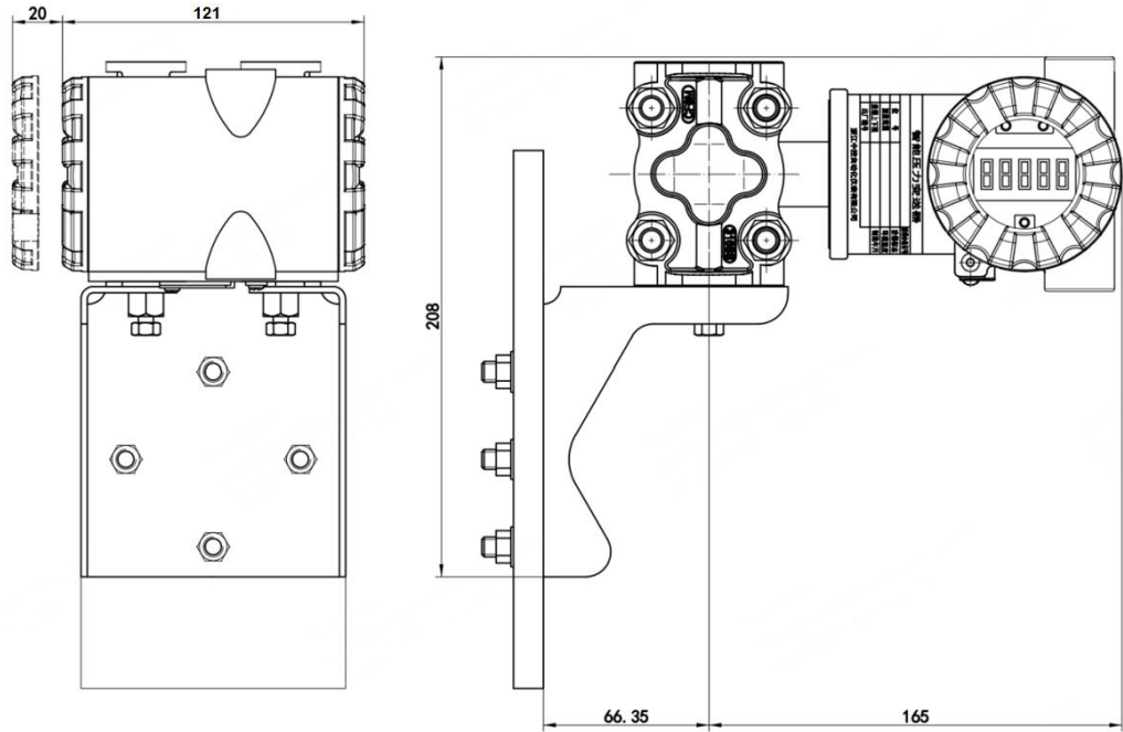
水平配管连接图（管装平支架）
