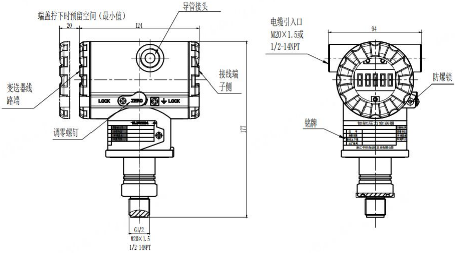
常规螺纹口示意图:
