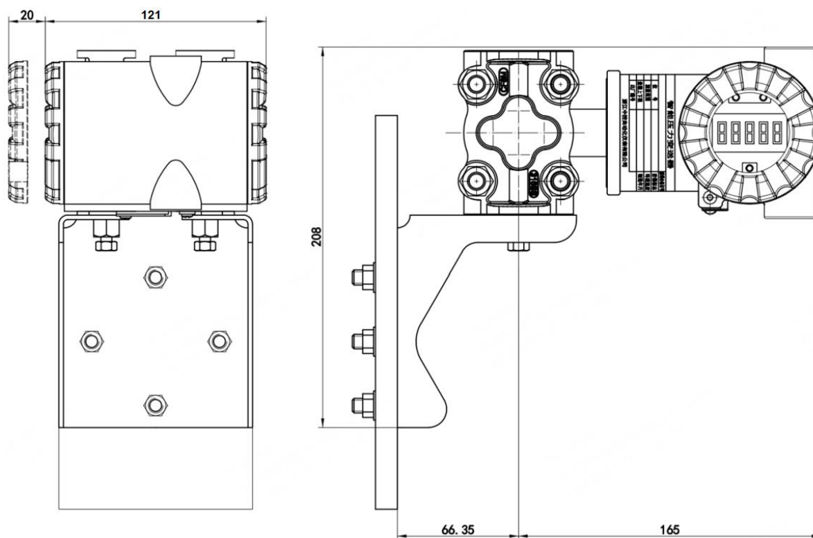
垂直配管连接图（板装弯支架）
