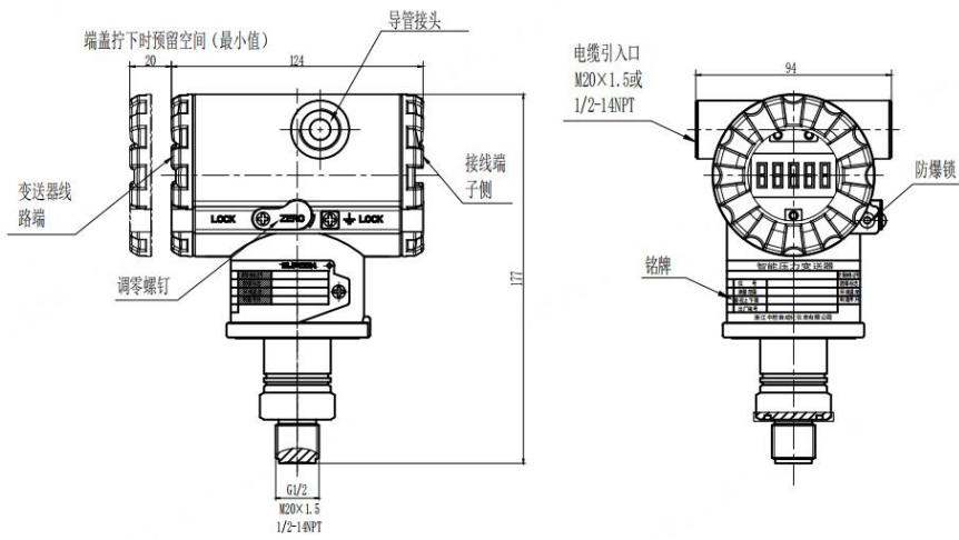
常规螺纹口示意图:
