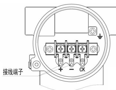
端子侧接线图
