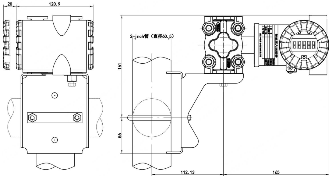
垂直配管连接图（管装弯支架）
