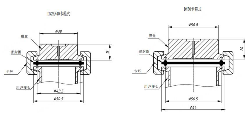
卫生型接口示意图:
