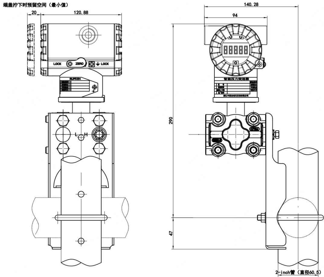
水平配管连接图（管装平支架）
