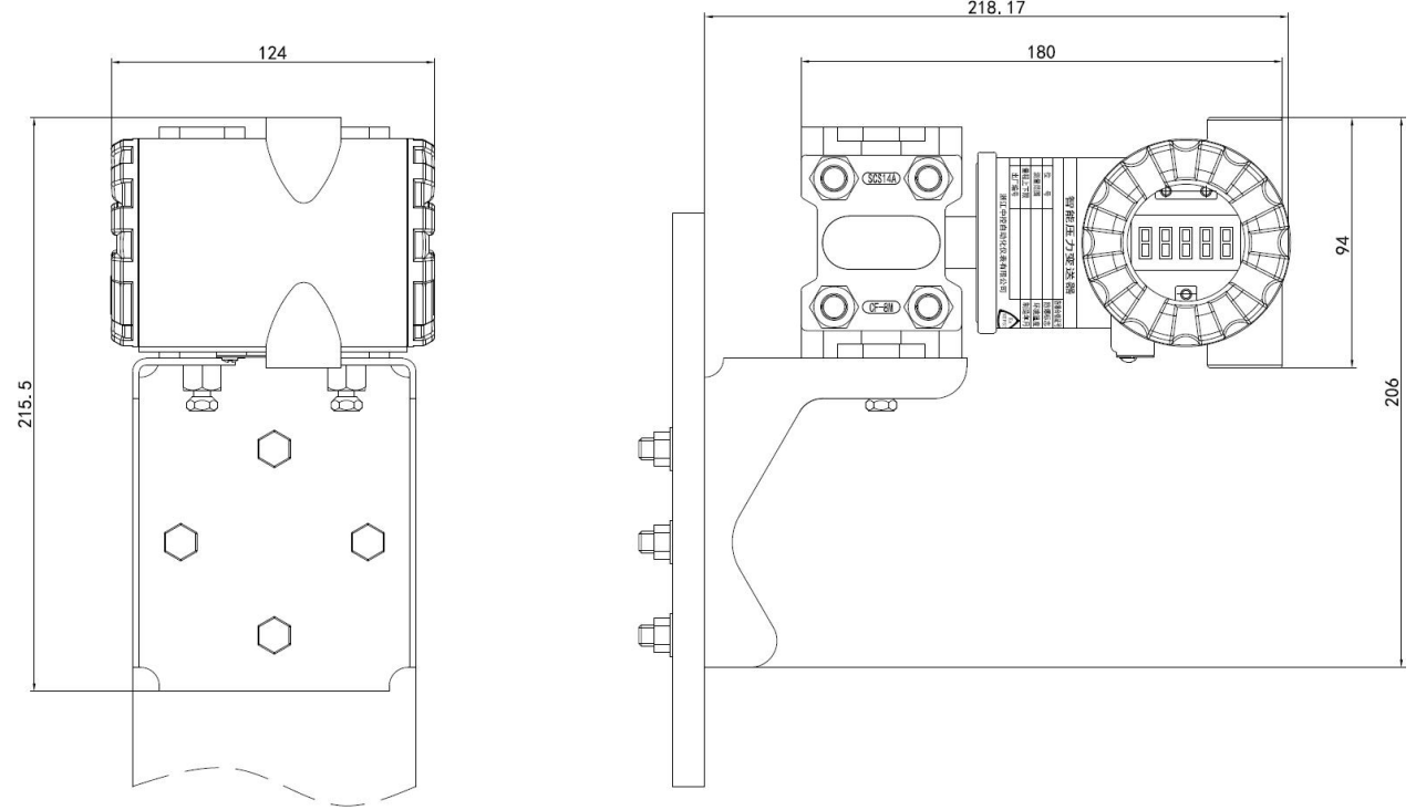
垂直配管连接图（板装弯支架）
