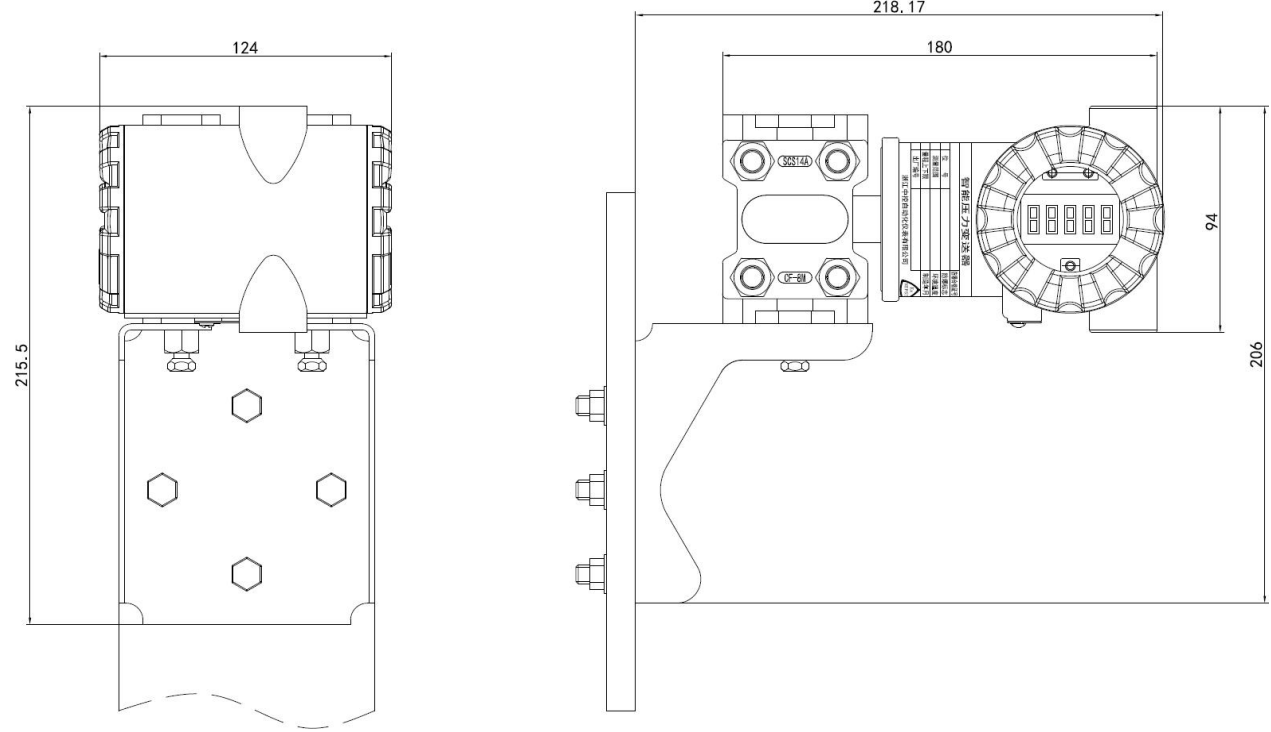
垂直配管连接图（板装弯支架）
