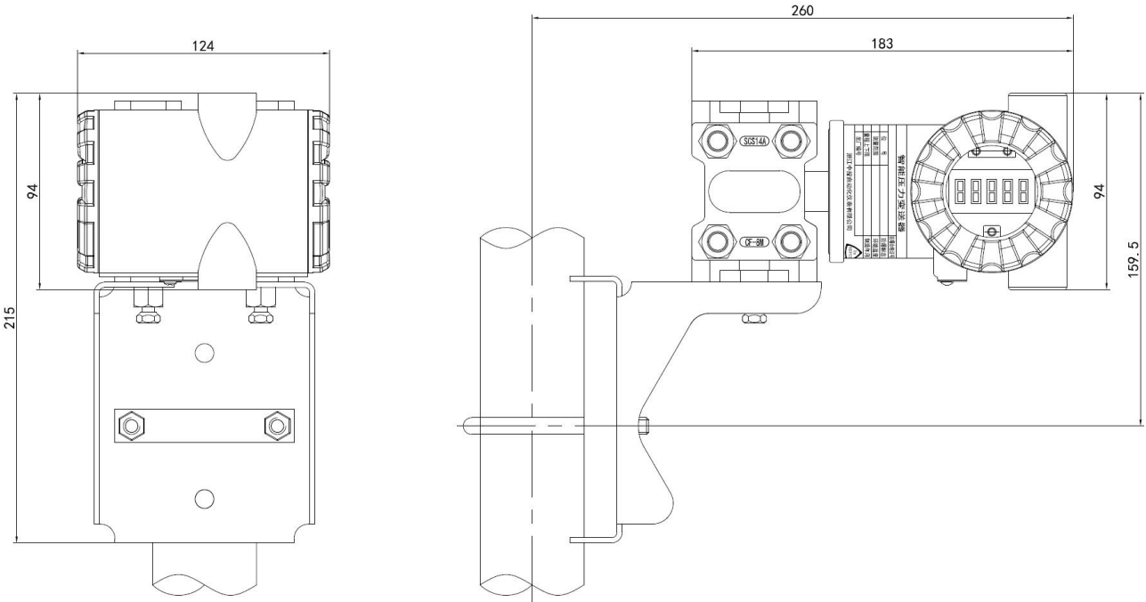
垂直配管连接图（板装弯支架）
