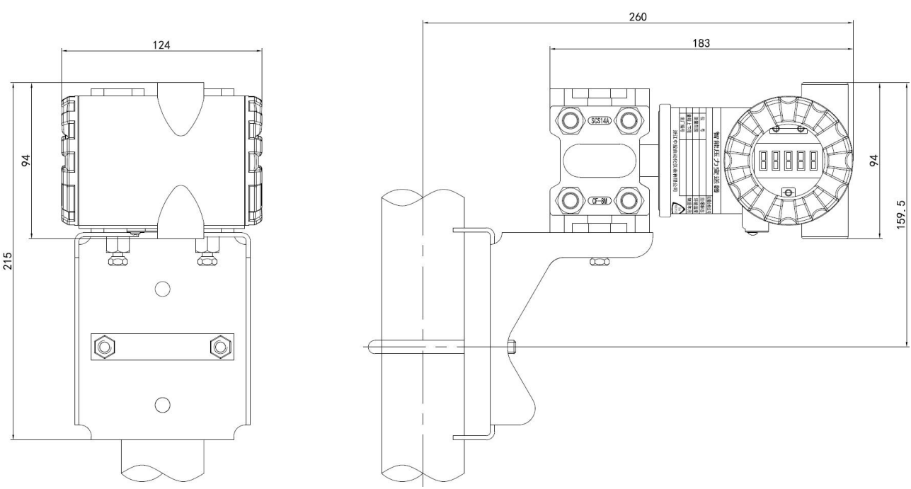
垂直配管连接图（管装弯支架）
