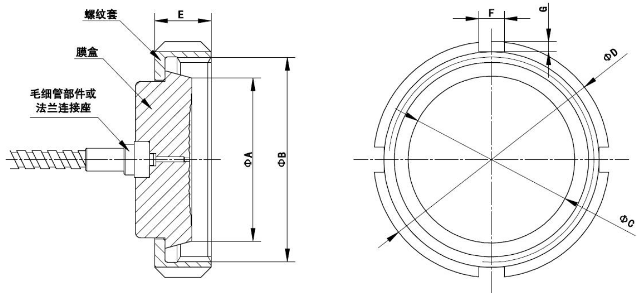
外形尺寸图（单位：mm）
